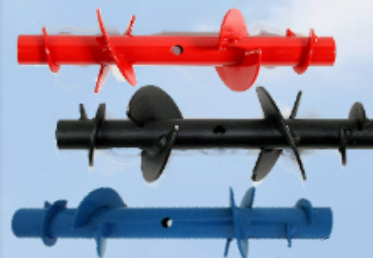
施肥排出量の目安 オーガー畦幅 75cmの場合 青 80~350kg/ha 赤 160~700kg/ha (NC標準) 黒 400~900kg/ha (NG標準)
